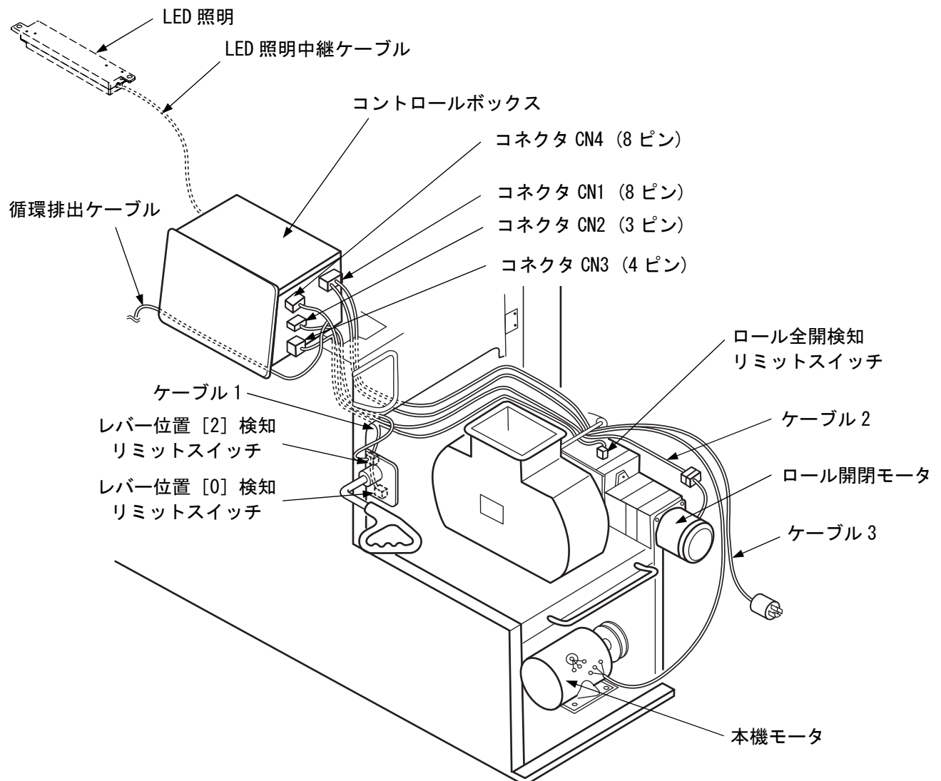
図 5 電装部品の構成
