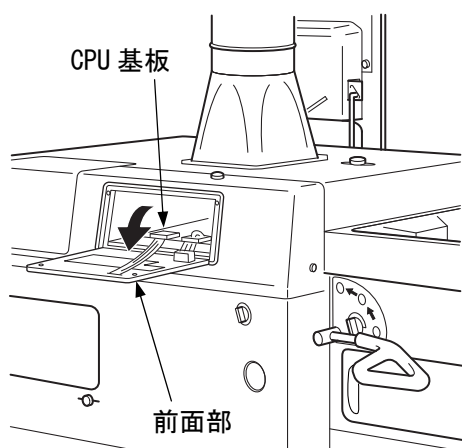
※CPU 基板を上から見た図
