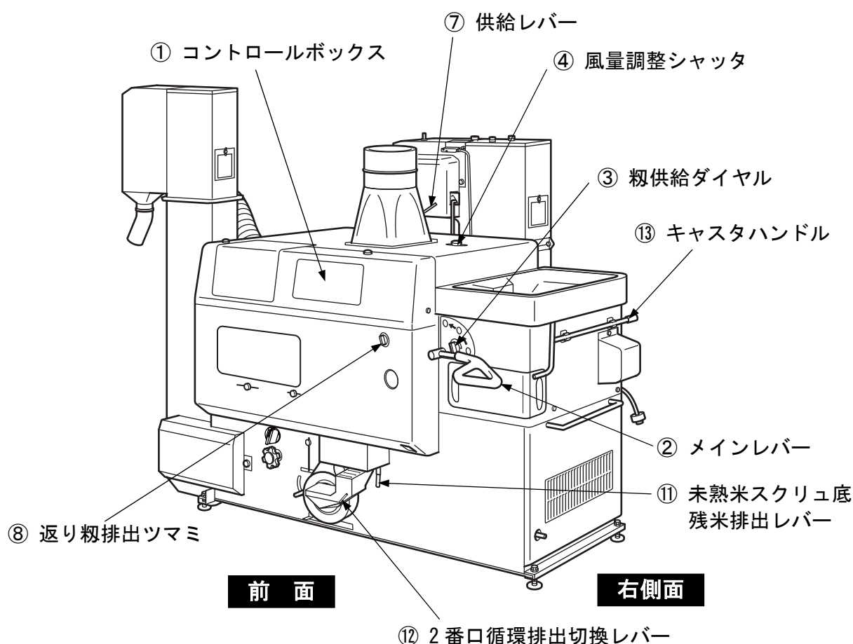
図 7 機械操作箇所 (1)
