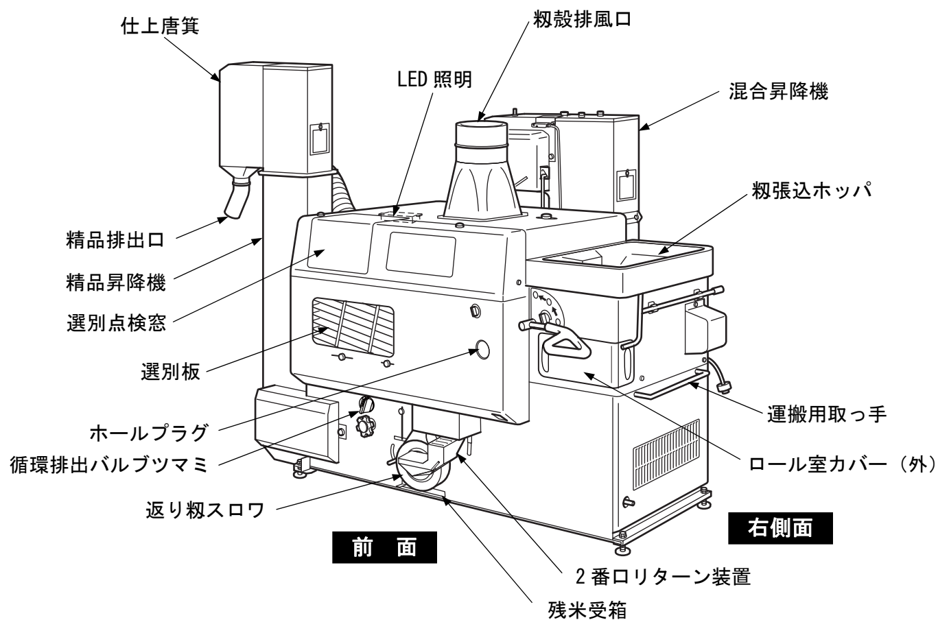
図 3 機械全体図 (1)
