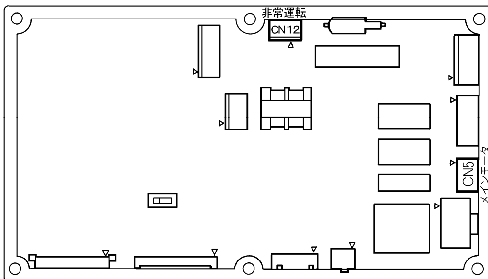
※CPU 基板を上から見た図
