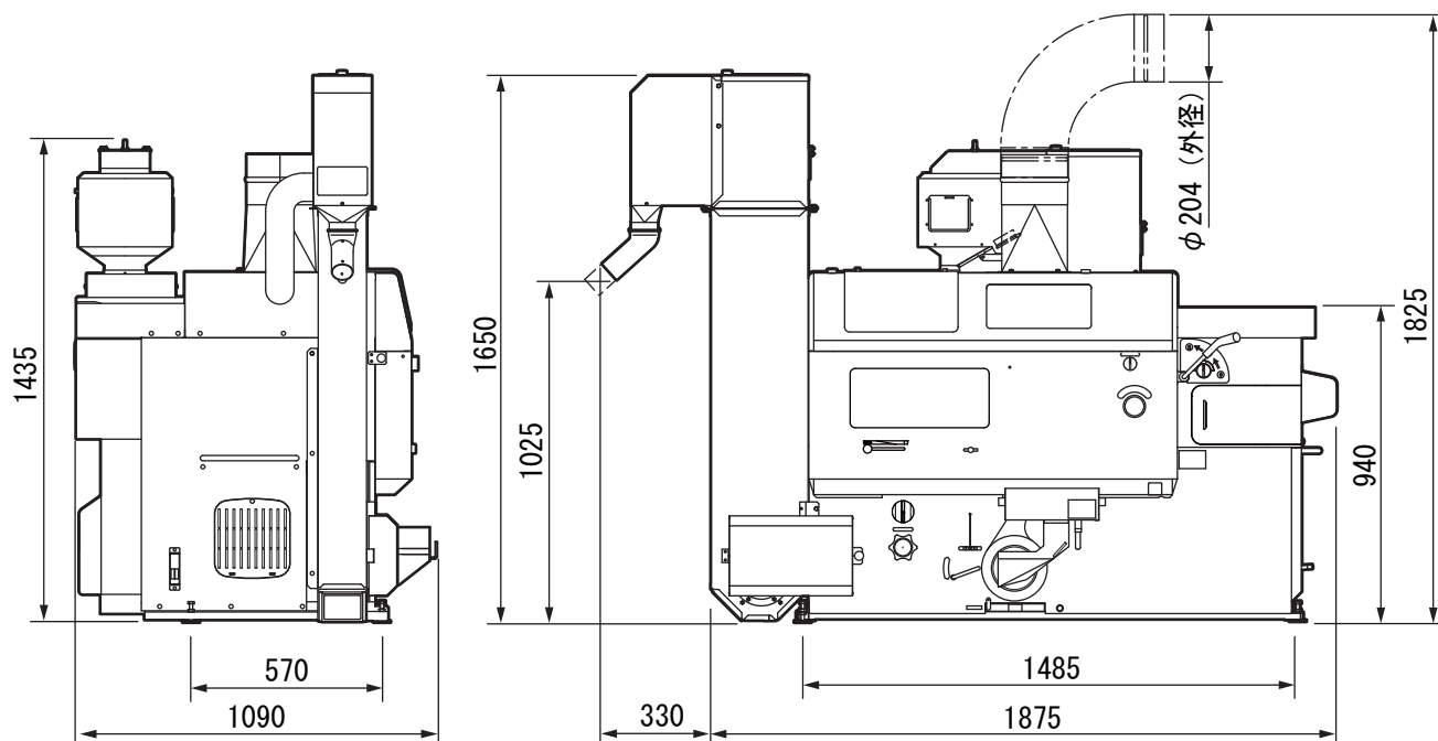
図 9 機体寸法
